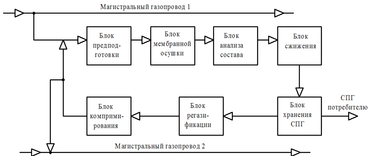
Рисунок 1 - Принципиальная схема экспериментальной СПГ-установки
